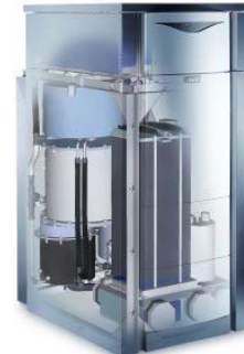
Caldaia con celle a combustibile della Vaillant
